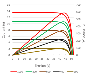
Courbes courant-tension et puissance-tension (580W)
